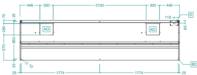
Boven aanzicht
